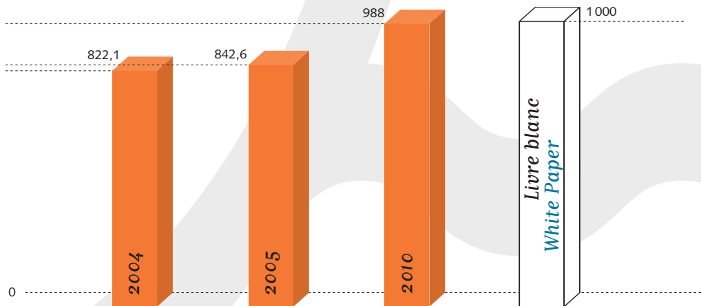
4 Comparaison de la tendance actuelle avec les objectifs du Livre blanc pour la production d'électricité (en MWe) Comparison between current trend and White Paper objectives for electricity production (in MWe)
